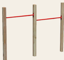
4. WINNETOO Spielreck* Material: Europ. Lärchenholz, Breite: 203, Höhe: 155, Pfosten: 88 x 88 mm (ohne Boden- anker), Pfostenköpfe abgeschrägt, mit Nut zur Aufnahme der Stangenhalterung, Reckstangen aus verzinktem Stahl, lackiert, Stangenhöhe variabel montierbar Art.-Nr. 1246 129,-
