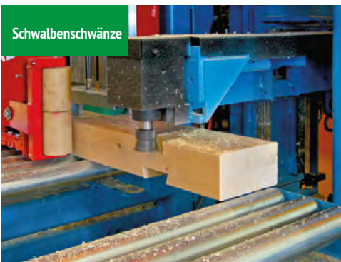
Schwalbenschwanz am Schifter
