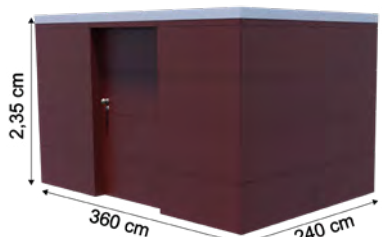
Art.-Nr. HPG15R
