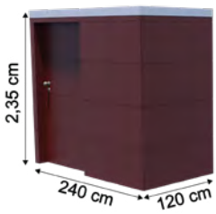
Art.-Nr. HPG05R
